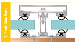
Universalprofil oben und unten, Distanzstück, Klemmdeckel (optional)
