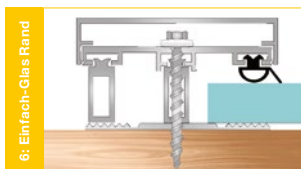
Auflagegummi unten, Universalprofil oben, Distanzstück, Klemmdeckel (optional)
