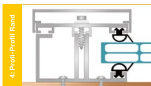
Randprofil unten, Universalprofil oben, Klemmdeckel (optional)
