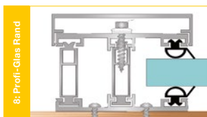
Universalprofil oben und unten, Distanzstücke, Klemmdeckel (optional)
