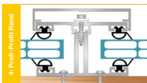
Mittelprofil unten, Universalprofil oben, Klemmdeckel (optional)
