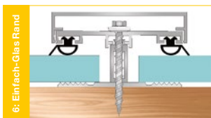
Auflagegummi unten, Universalprofil oben, Klemmdeckel (optional)
